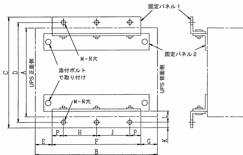
床面加工図
