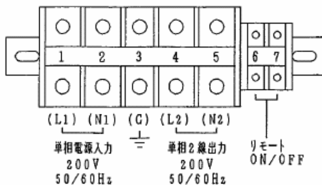
図 6.2 入出力端子台
