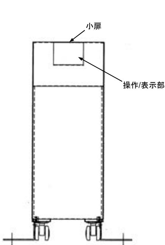
正面図
