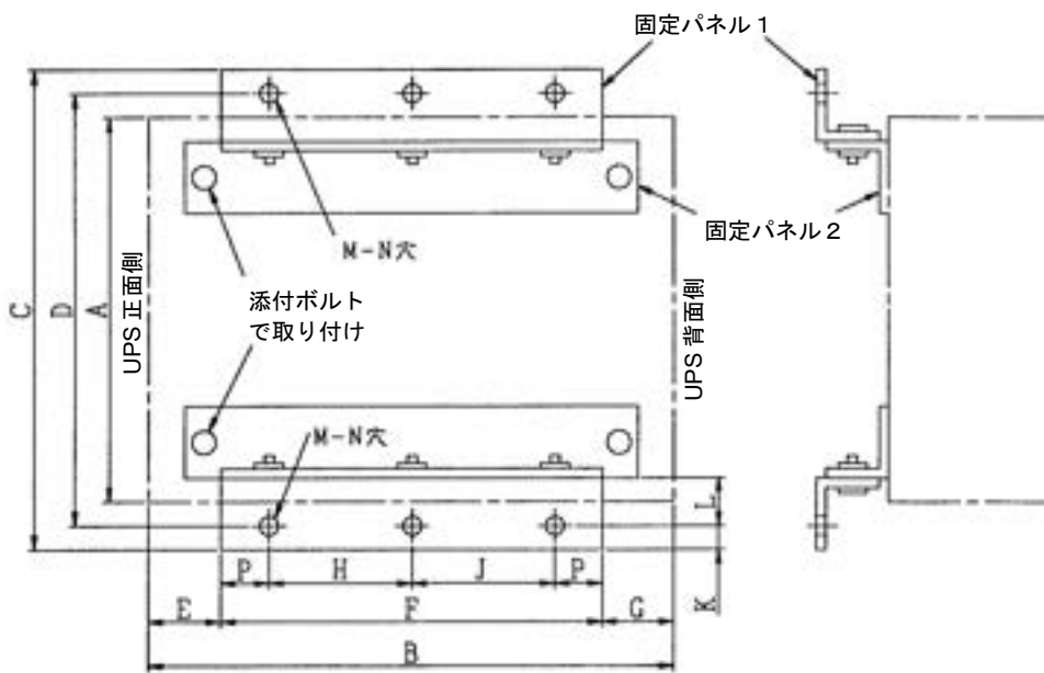
床面加工図
