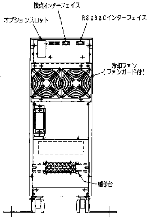
背面図
