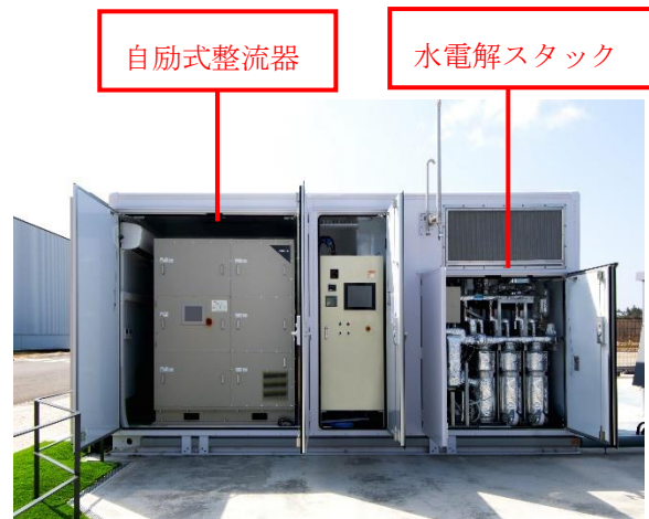
水電解装置(内部)
