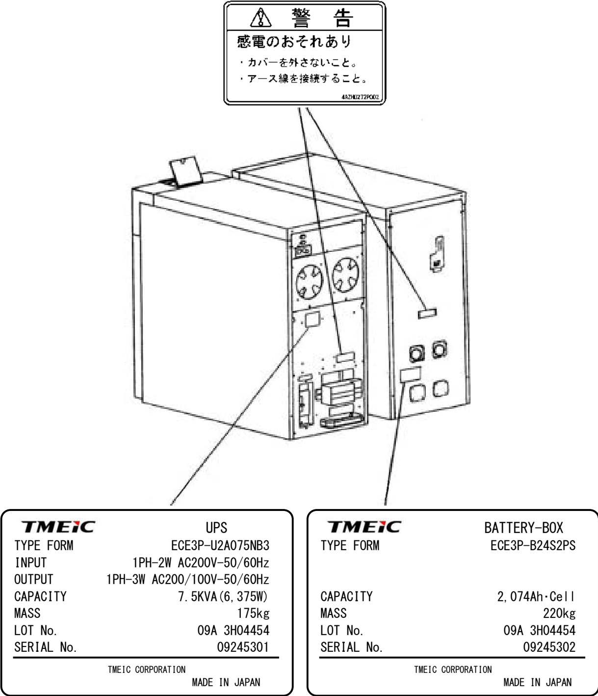
図2. 3 背面側 安全ラベル貼付位置(7.5KVA 力率 0.7 時の 30 分延長の例)
